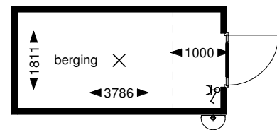
Begane grond
