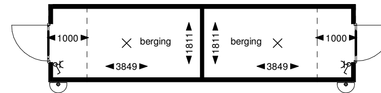
Begane grond
