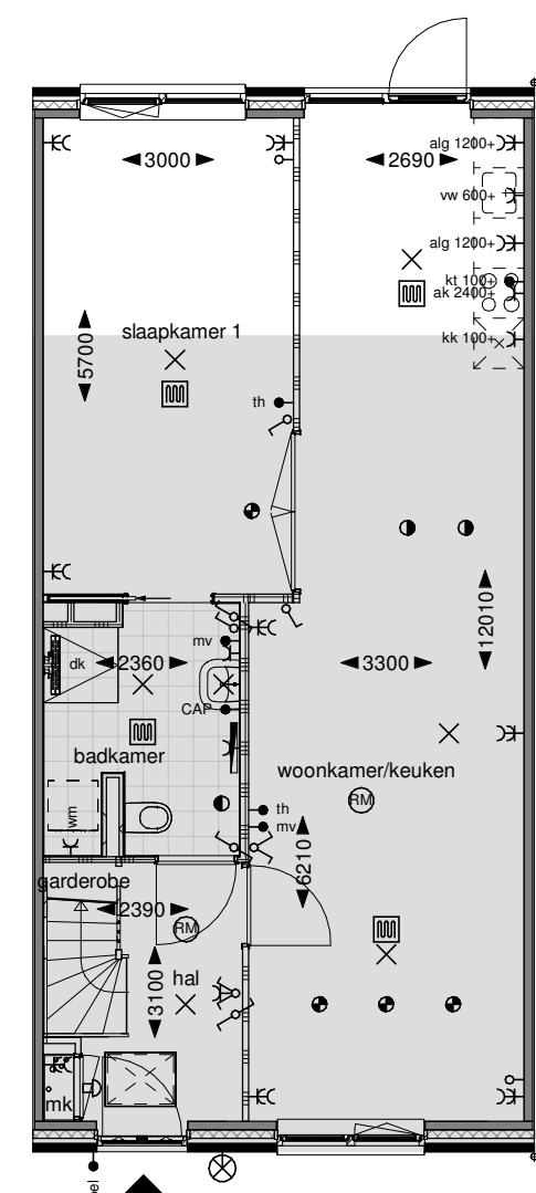
Begane grond
