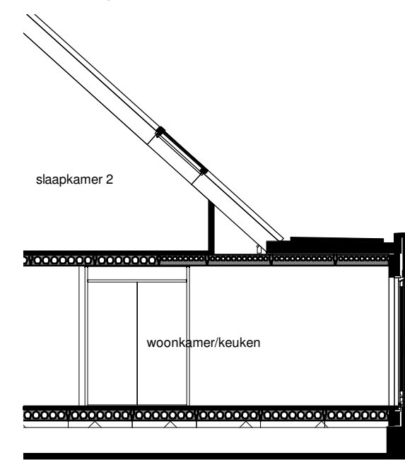
Doorsnede
