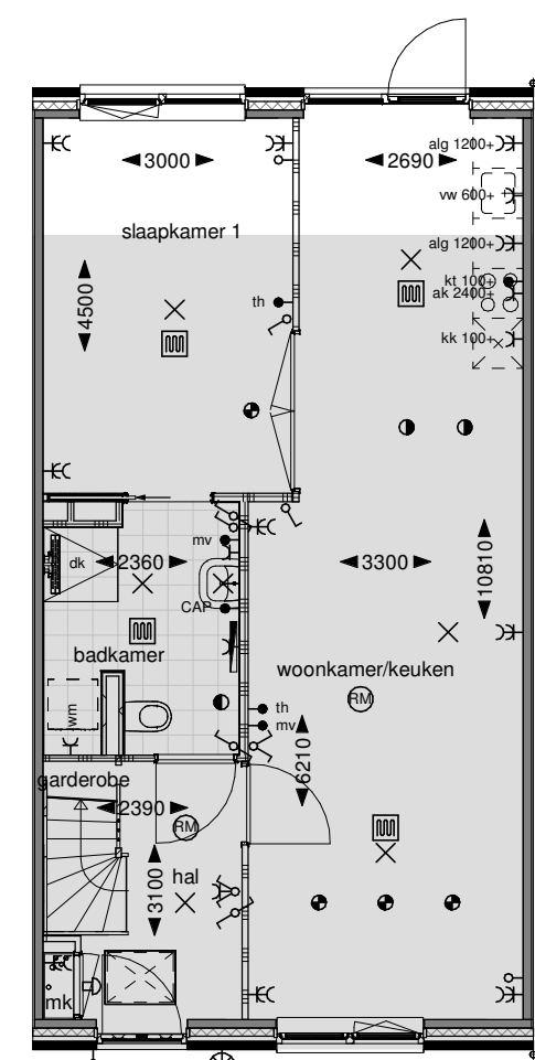
Begane grond
