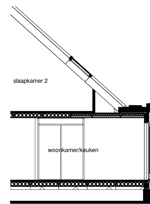
Doorsnede
