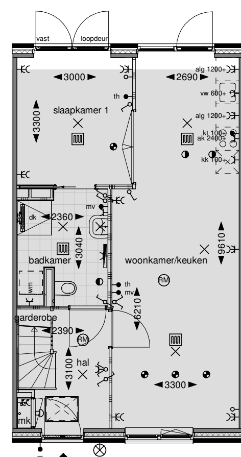
Begane grond
