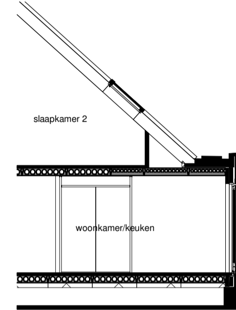
Doorsnede
