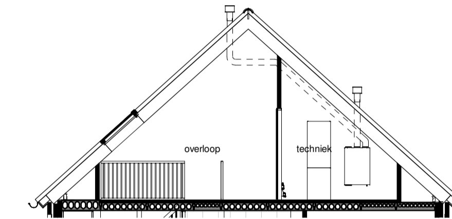
Doorsnede
