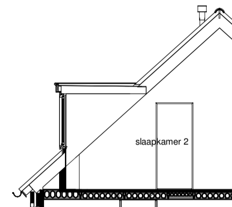
Doorsnede
