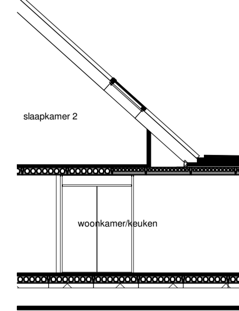
Doorsnede
