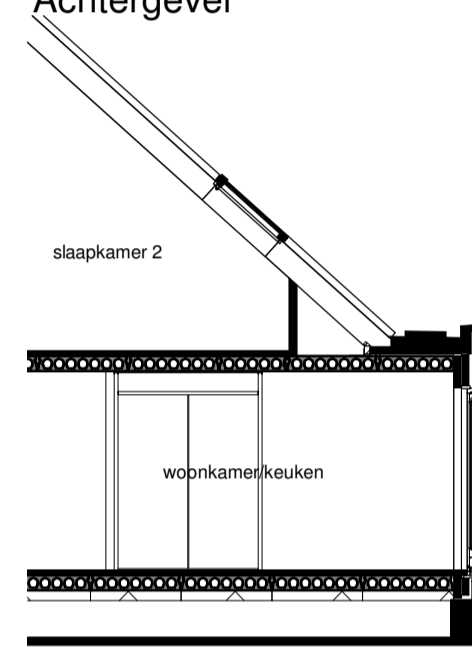
Doorsnede
