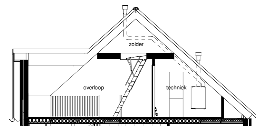
Doorsnede
