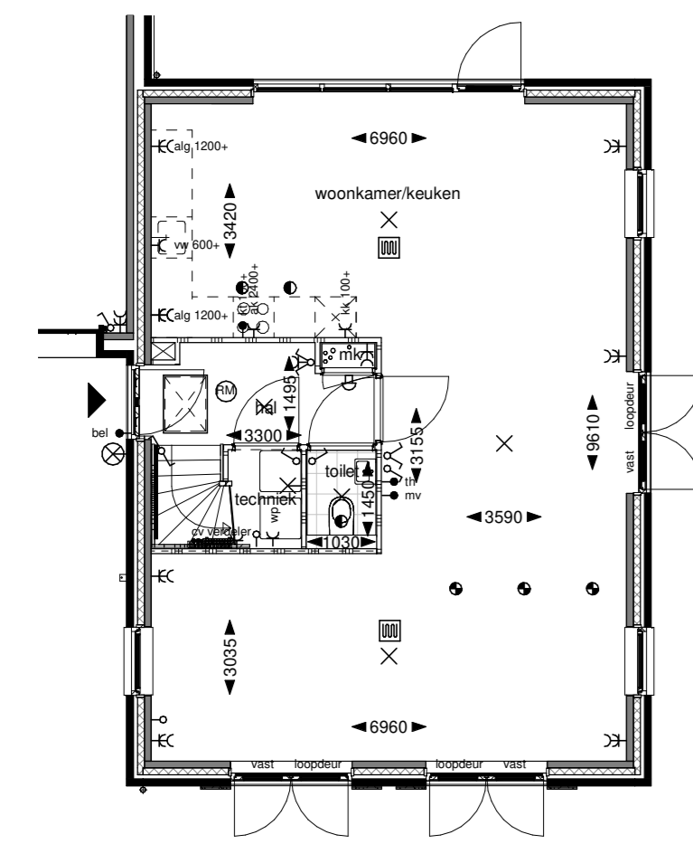
Begane grond
