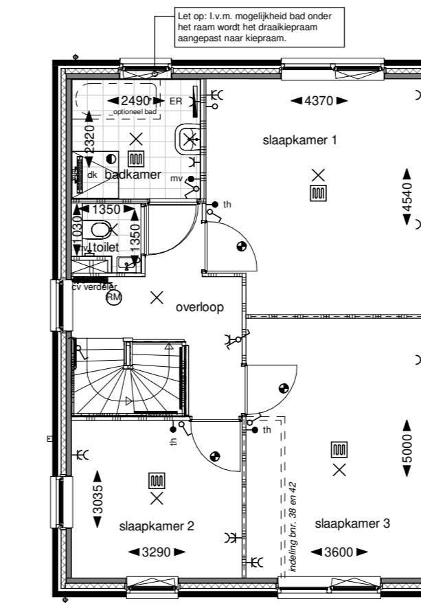
Eerste verdieping
