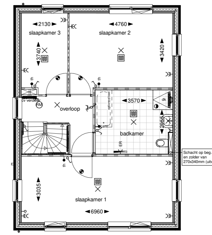
Eerste verdieping
