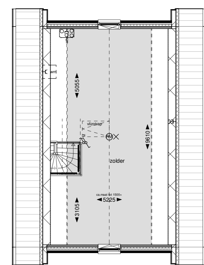
Tweede verdieping
