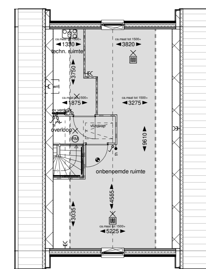
Tweede verdieping
