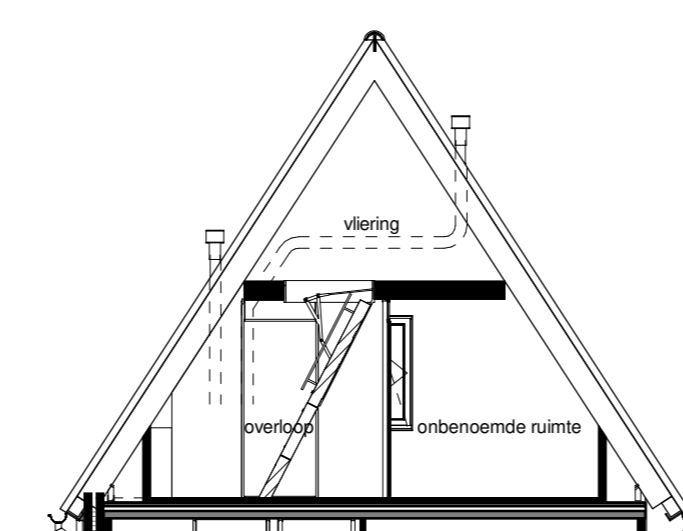
Doorsnede
