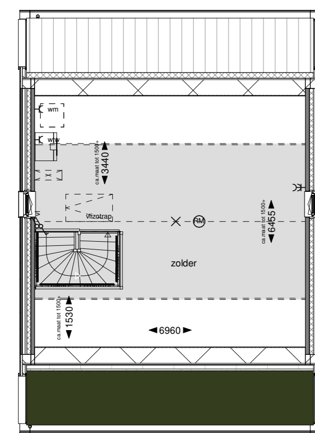
Tweede verdieping
