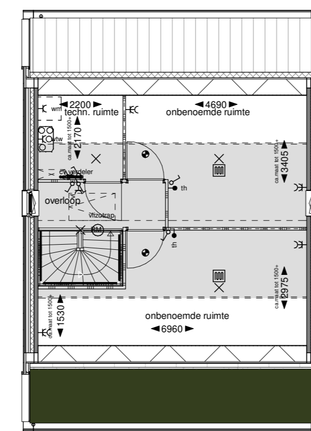
Tweede verdieping
