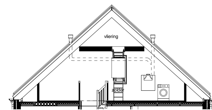
Doorsnede
