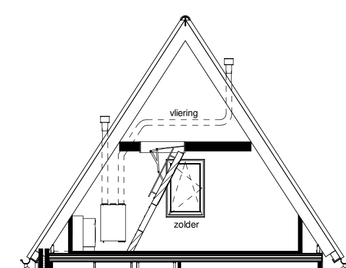
Doorsnede
