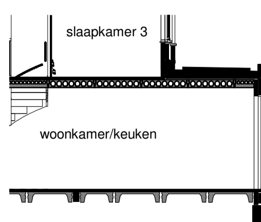
Doorsnede
