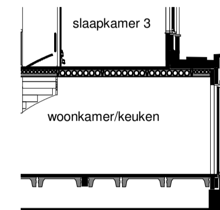
Doorsnede
