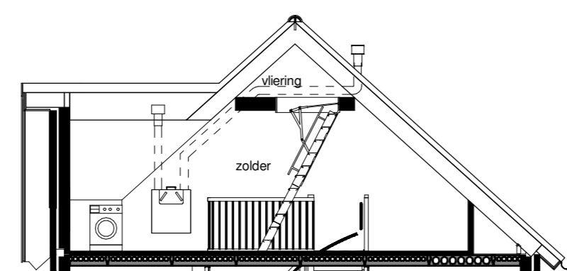
Doorsnede
